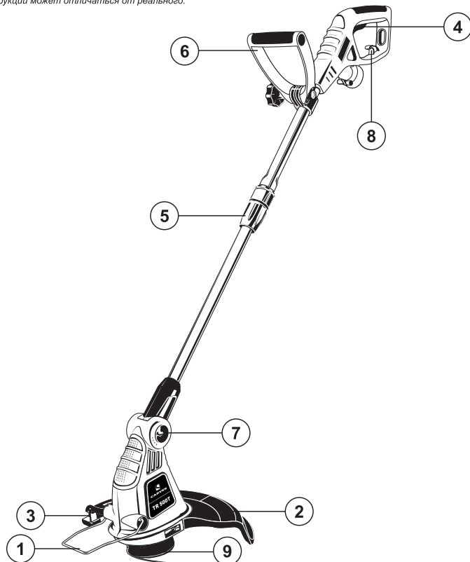
Рис.2. Расположение основных элементов электротриммера:
