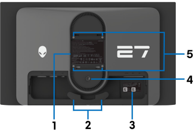
Вид сзади - монитор без стойки
