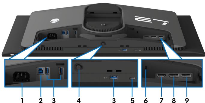
Вид монитора сзади и снизу без стойки
