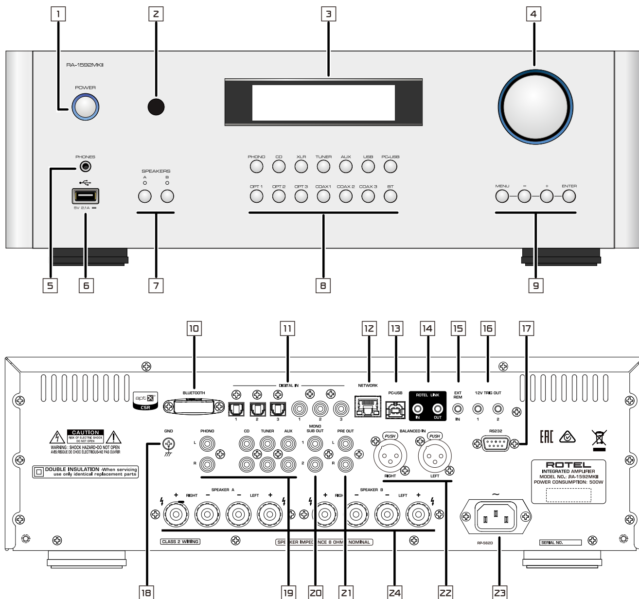
Figure 1: Controls and Connections Commandes et Branchements Bedienelemente und Anschlüsse Controles y Conexiones Bedieningselementen en aansluitingen ontrolli e connessioni Kontrollor och anslutningar Органы управления и разъемы
